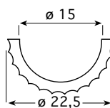
C COL3244 Mezzo capitello dorico 37 x 18,5 x H. 30 cm Half doric capital 14 9/16" x 7 5/16" x H. 11 13/16"
