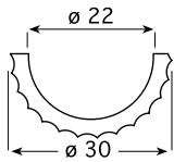
C COL3354 Mezzo capitello ellenico 54 x 23,5 x H. 17 cm Half hellenic capital 21 4 / 16 " x 9 4 / 16 " x H. 4 5 / 16 "
